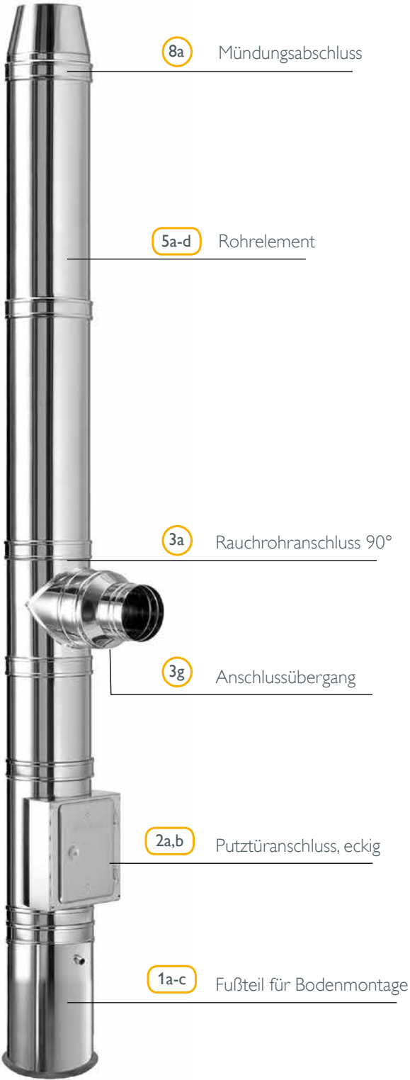
Bodenmontage
