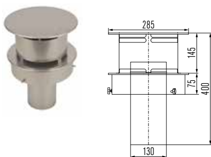
Mündungsabschluss mit Regenhaube und Windabweiser
