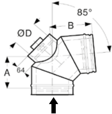
Bogen 85° mit Revisionsverschluss für Öl, Gas
