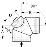
Bogen 90° mit Revisionsverschluss für Öl, Gas
