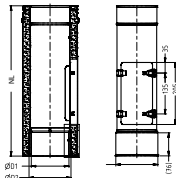
Rußtopf
