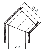
LB90 – Bogen 45°
