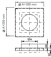
LB90 – Abdeckplatte
