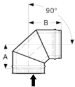
Bogen 90° mit Reinigungsöffnung, flach
