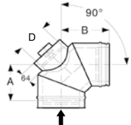
Bogen 90° mit Revisionsverschluss für Öl, Gas
