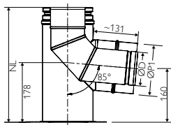
Rauchrohranschluss 85° mit Luftansaugung
