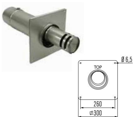
Horizontale Mündung 100 exzentrisch mit Abdeckblende eckig 300
