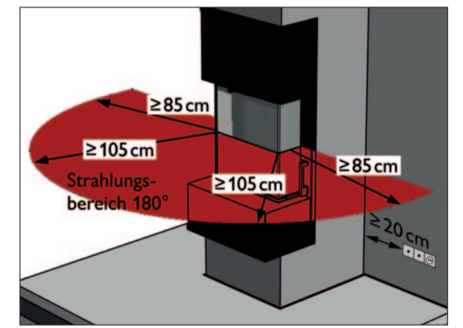
Strahlungsbereich für KINGFIRE GRANDE SC
