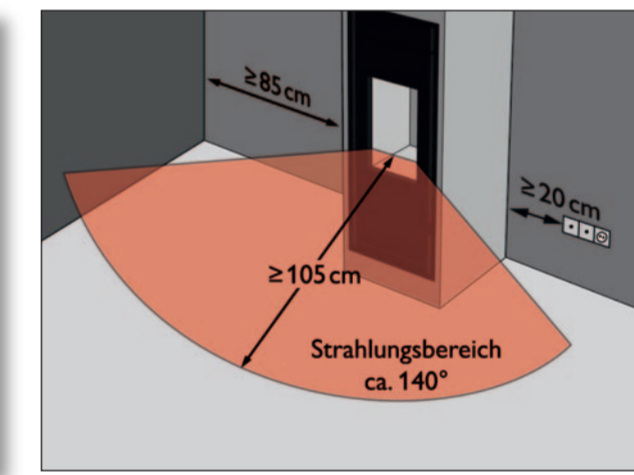
Strahlungsbereich für KINGFIRE CLASSICO S, RONDO SC, LINEARE SC
