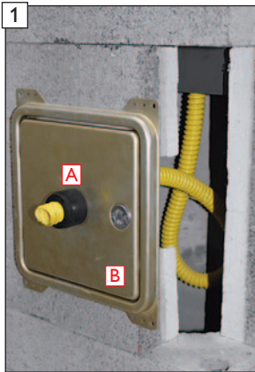
Lieferzustand ab Werk mit BlowerDoor Kondensatblendentür (B) und in der Dichtung (A) eingedrehtem Siphonschlauch.
