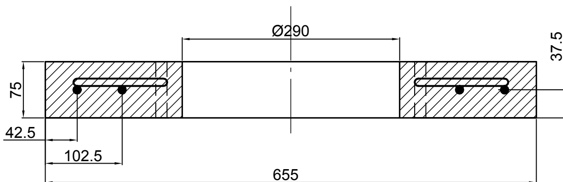
Snit A-A
