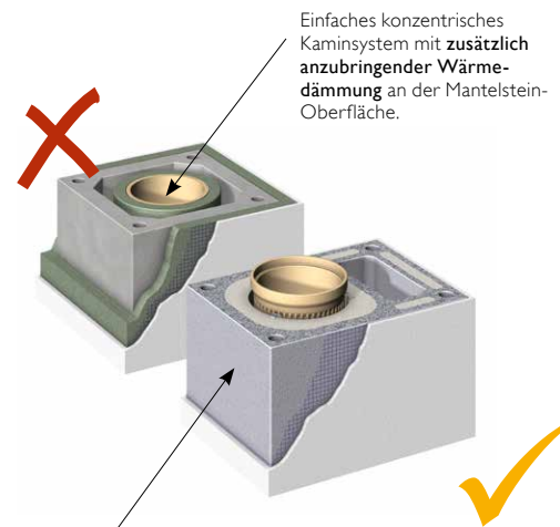
ABSOLUT TL mit Compound-Mantelstein, integrierter, werkseitiger Dämmung und gedämmtem Thermo-Luftzug.
