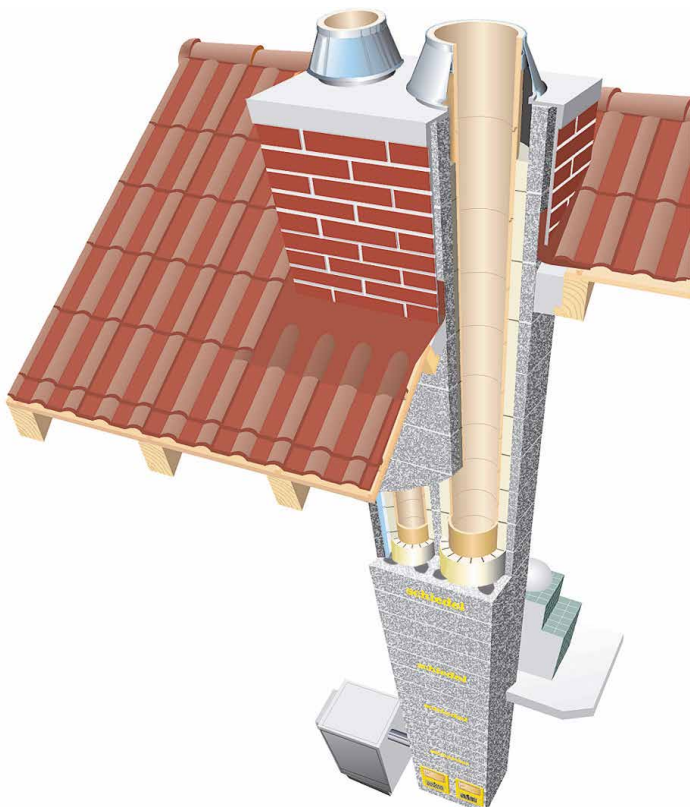
Schiedel Fertigfuß – der erste Kaminmeter
