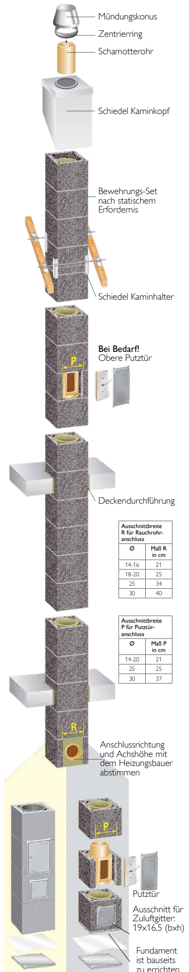
Optional: Installationszug - für nicht brennbare Leitungen (Photovoltaik,...)
