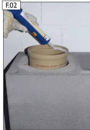
RAPID-fugendicht satt auftragen.
