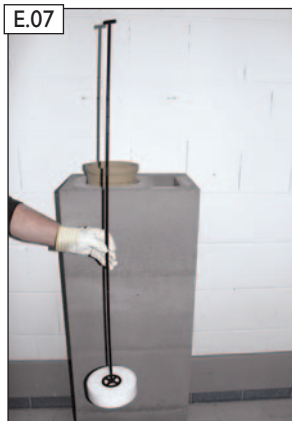
E.07 Gesamtansicht fertig zusammgebauter Fugenglätter.
