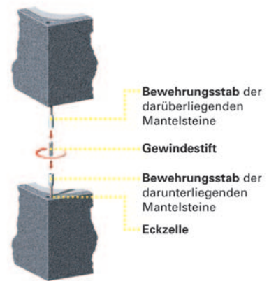
Bild 2 - Verschraubung
