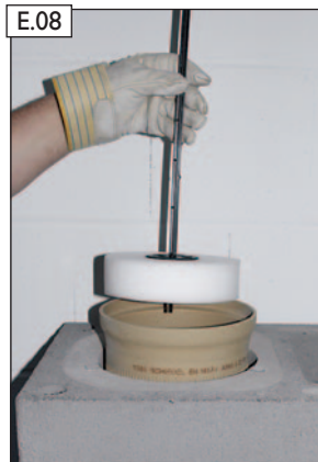
E.08 Reste von RAPID-fugendicht mit Fugenglätter abstreifen.
