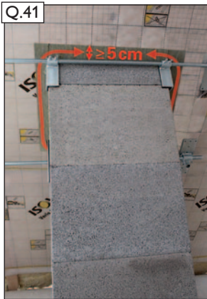
Q.41 Fertigansicht mit ausgedämmtem Dachdurchgang gem. FeuVo der Länder.
