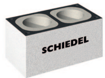
Thermotrennstein: Integrierte Schaumglas-Dämmschicht zur Unterbrechung der Wärmelängsleitung
