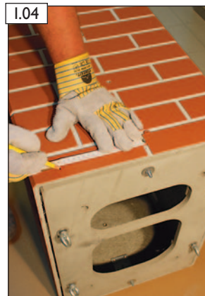
Ermittelte Abmessungen C des Mantelsteins mittig auf den Stülpkopf übertragen.
