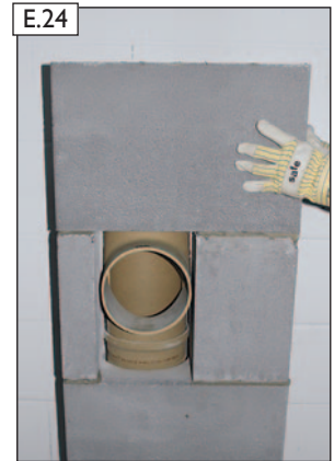
Nächsten Mantelstein versetzen.
