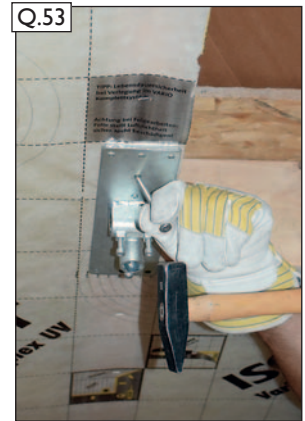
Q.53 Sparrenhalter mit Kamm-nägeln (E) ausnageln.
