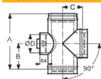
T-idom 90 fokos N1 vizsgáló nyílással
