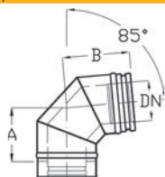
Könyök 85 fokos N1 vizsgálónylással
