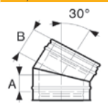
Könyök 30 fokos
