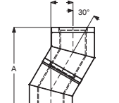
Könyök 30°
