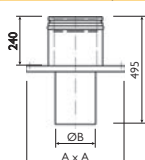
Talpelem kéménytoldáshoz ABS-ICS25
