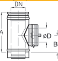
Vizsgálónylásos elem N1 (rövid)
