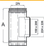
Tisztítóajtós elem
