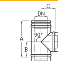
T-idom 90 fokos
