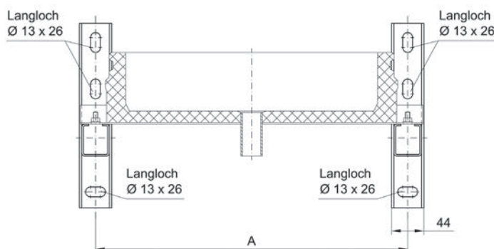
Méret az a 325-től a 475-ös típusok esetén
