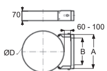
Állítható falbilincs 60-100
