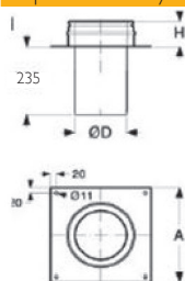
Talplelem kéménytoldáshoz UNI-ICS50
