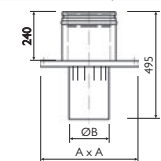
Talpelem kéménytoldáshoz UNI-ICS25
