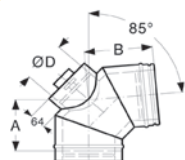
Könyök 85 fokos N1 vizsgálónylással
