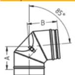
Könyök 85 fokos vizsgálónylással
