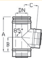
T-idom 85 fokos
