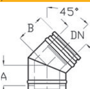
Könyök 45 fokos
