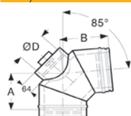
Könyök 85 fokos N1 vizsgálónylással
