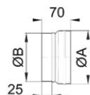
Adapter huzatszabályozóhoz
