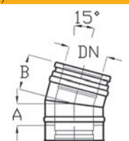
Könyök 15 fokos
