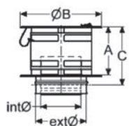
Esővédő gallér
