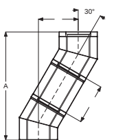
Könyök 30° csőelemmel
