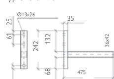
Falkonzol hosszú (pár)
