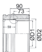
Adapter (rövid)
