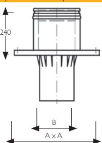
Talplelem kéménytoldáshoz UNI-ICS50
