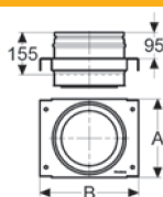
Közbenső támasz
