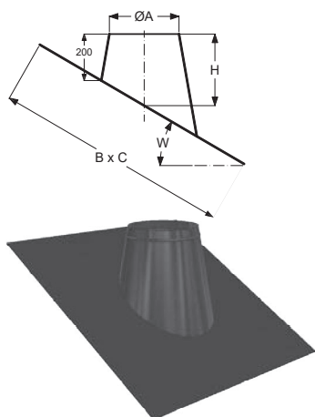
Tetőátvezető, vörös waka-flex-szel
