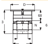
Esővédős kéményfej záróelem
