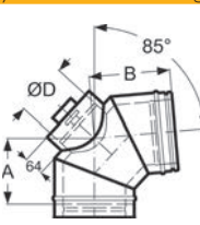
Könyök 85 fokos N1 vizsgálónylással
