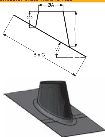
Tetőátvezető, fekete waka-flex-szel
