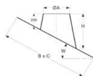
Tetőátvezető, fekete waka-flex-szel
