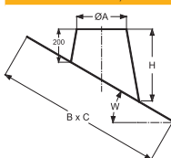
Tetőátvezetők, fekete waka-flexszel (INOX kúpos palást / fekete waka-flex)
