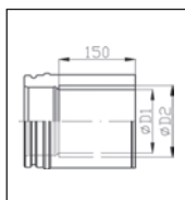
Adapter (hosszú)
