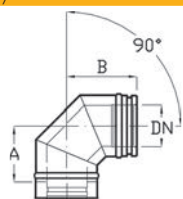
Könyök 90 fokos, vizsgálónylással
