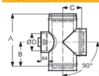
T-idom 90 fokos P1 vizsgáló nyílással
