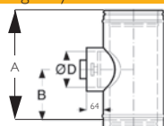
Vizsgálónyílásos elem P1
