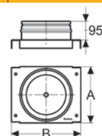
Közbenső támasz
