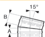
Könyök 15 fokos
