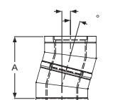
Könyök 15°
