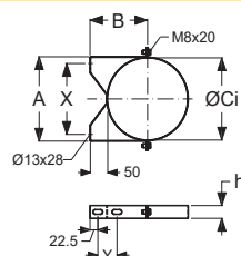
Erősített falbilincs
