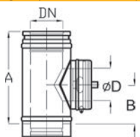
Vizsgálónyílásos elem P1 (rövid)
