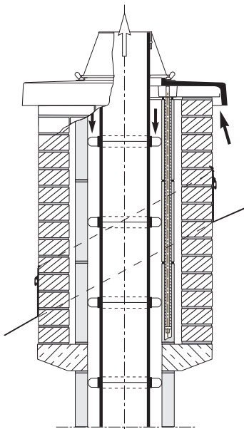
Körbefalazott fejkialakítás
