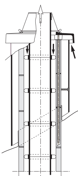
Hőszigetelt, vakolt fejkialakítás
