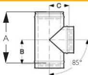
T-idom 85 fokos
