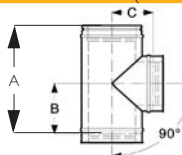
T-idom 90 fokos (rövid)
