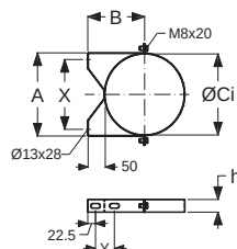
Erősített falbilincs
