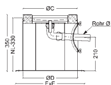
Talpelem padlószelészhez
