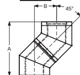
Könyök 45°
