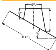
Tetőátvezetők, fekete wakaflaxszel (INOX kúpos palást / fekete wakaflax)
