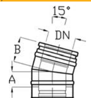
Könyök 15 fokos
