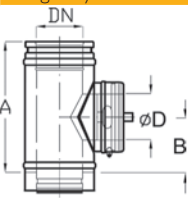
Vizsgálónylásos elem N1 (rövid)
