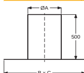
Tetőátvezető 0° (INOX)
