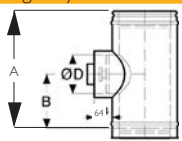
Vizsgálónylásos elem N1 (rövid)
