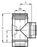
Vizsgálónyílásos elem, hátsófal
