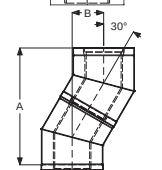
Könyök 30°
