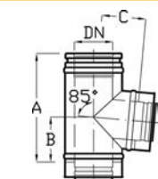
T-idom 85 fokos
