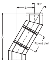
Könyök 30° csőelemmel
