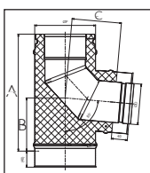
Talpas könyök 85° ICS25
