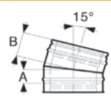
Könyök 15 fokos
