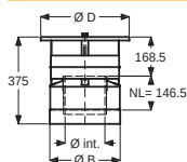
Esővédős kéményfej záróelem
