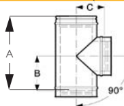
T-idom 90 fokos (hosszú)
