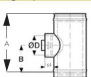
Vizsgálónylásos elem P1 (rövid)
