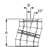
Könyök 15°
