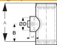
Vizsgálónylásos elem N1
