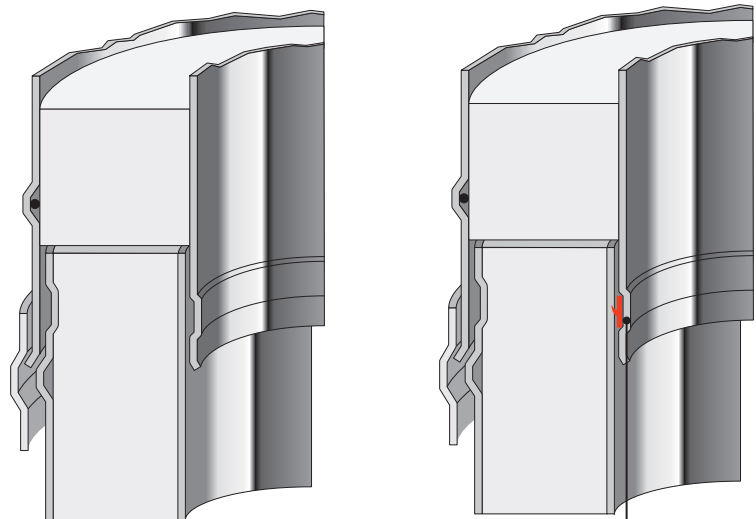
Ущільнювальна манжета для роботи з конденсаційними котлами або при надмірному тиску до 200 Па. Обмеження за температурою газів: до 200 гр.С
