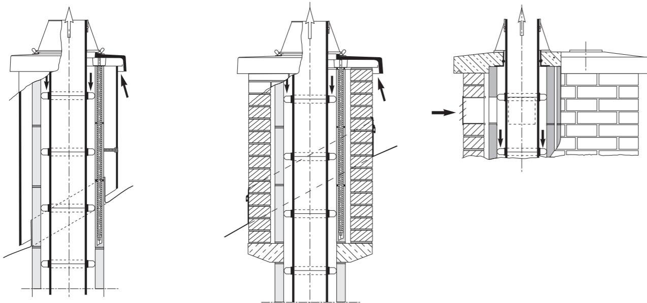
Hőszigetelt, vakolt fejkialakítás
