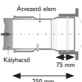
Füstcső-csatlakozó T-idomhoz, tömítő szalaggal
