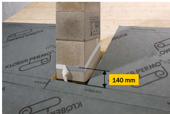
Nalepte obojstrannú butylovú lepiacu pásku na komínové teleso paralelne k strešnej rovine
