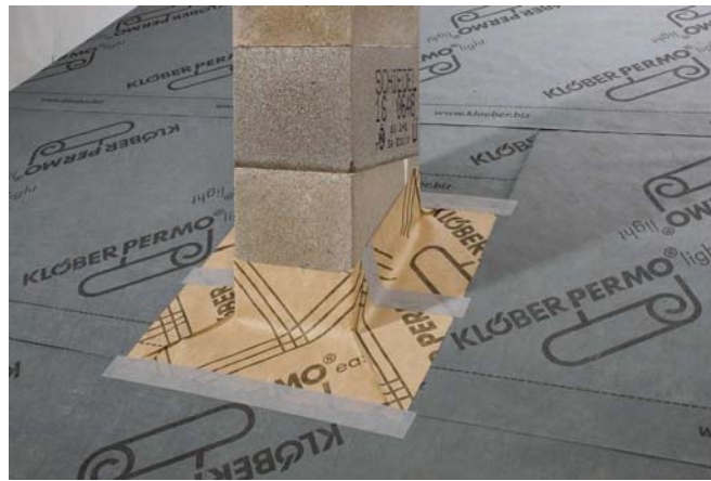
Rozložte vrchnú časť fólie, prilepte ju na pripravenú lepiacu pásku, z ktorej ste odstránili kryt lepej vrstvy. Prelepte páskou okraje fólie ako aj styky samotných fólií
