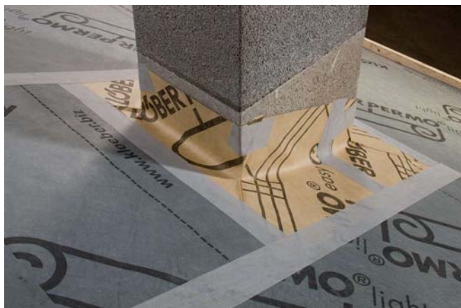
Rozložte spodnú časť fólie, prilepte ju na pripravenú lepiacu pásku, z ktorej ste odstránili kryt lepej vrstvy
